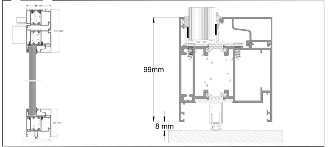
Kesit
